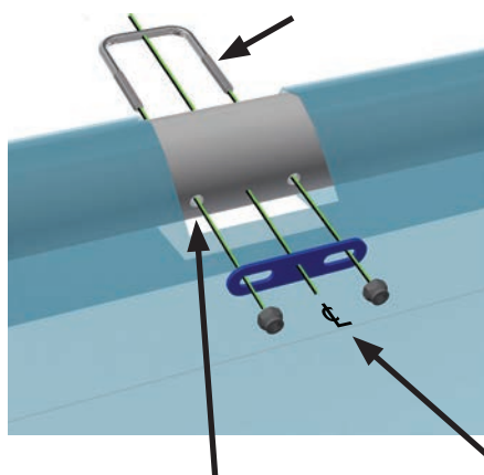
U-Bolt
